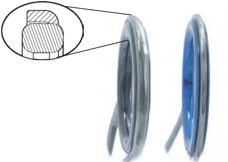
DV guide frame SV guide frame
